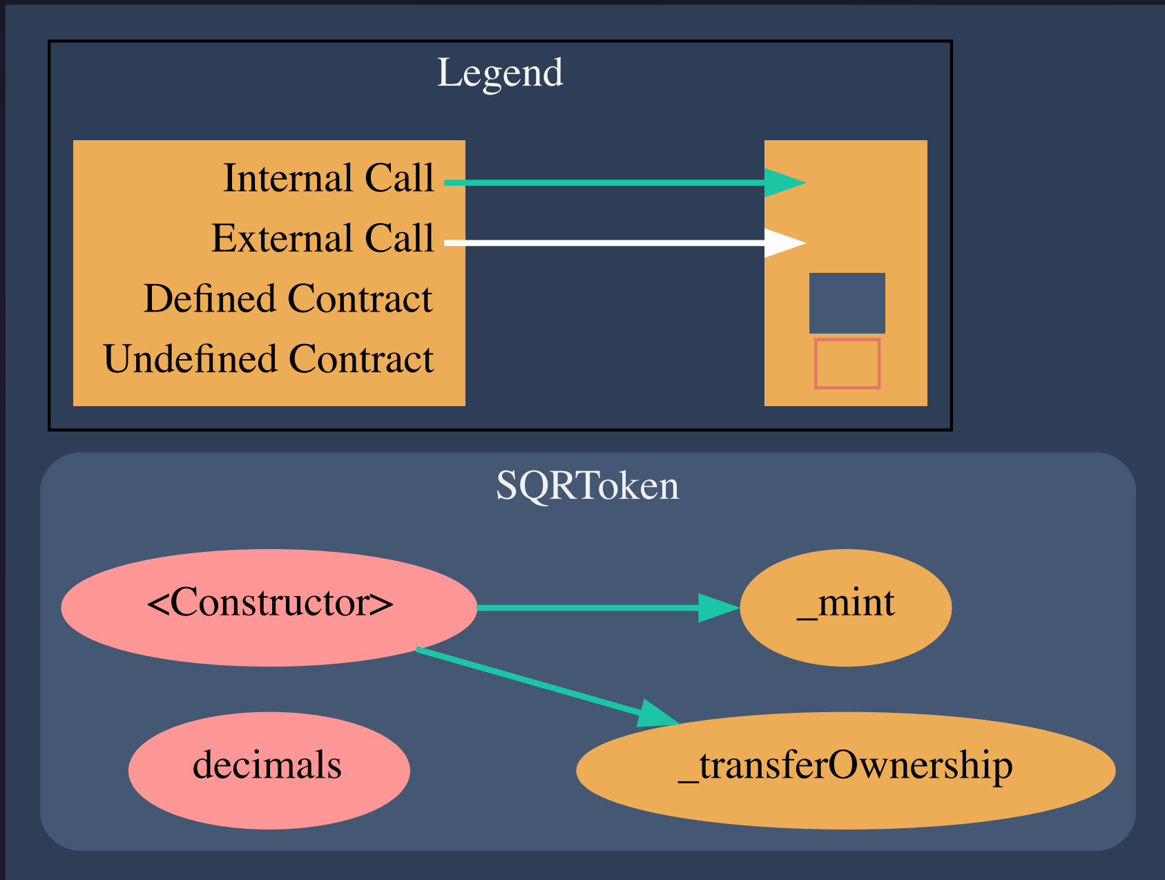
pic.1.1 SQRToken
